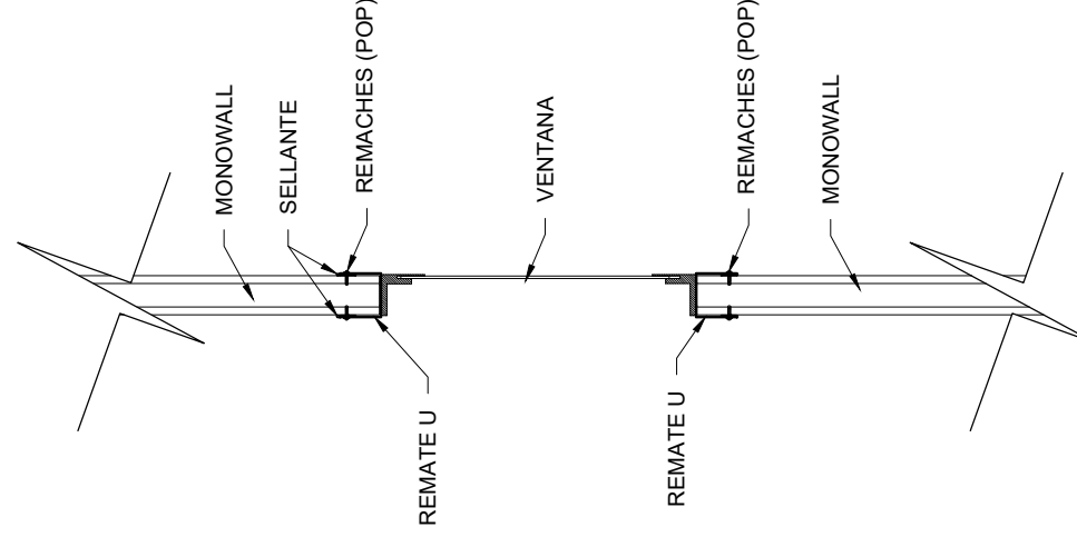
VISTA CORTE
